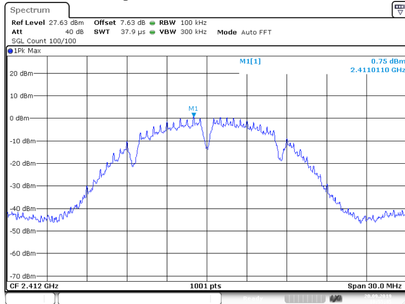
Band Edge NVNT 802.11b 2412MHz Ant1 Ref
