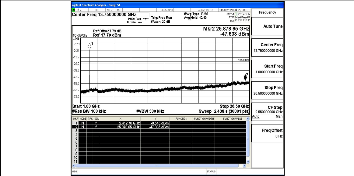
11B_Ant1_2412_1000~26500
