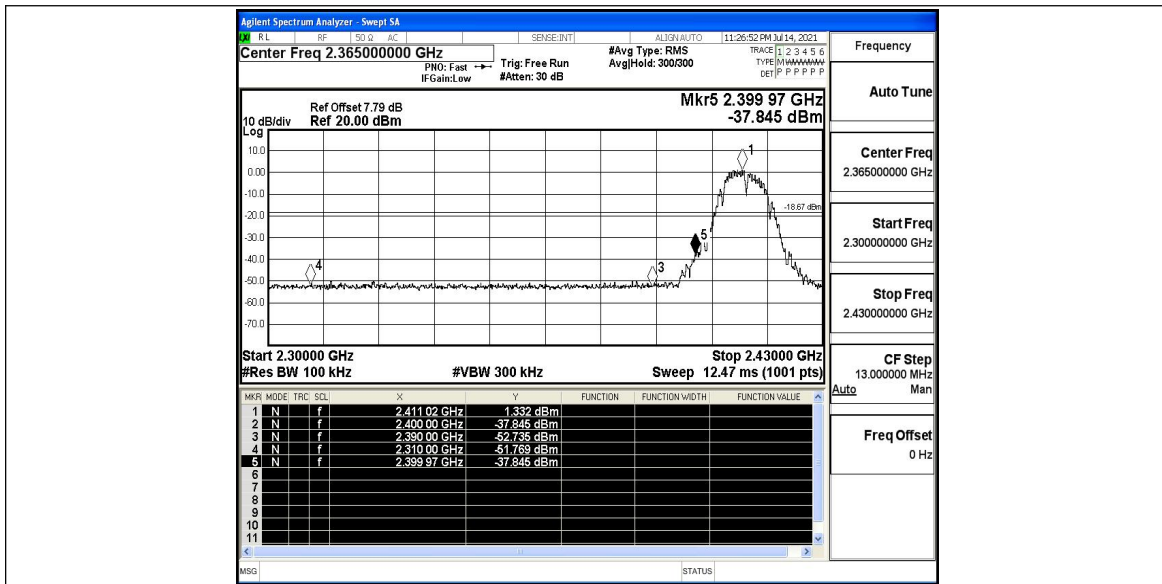
11B_Ant1_Low_2412
