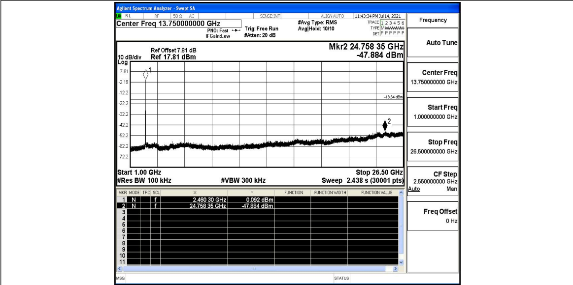
11B_Ant1_2462_1000~26500
