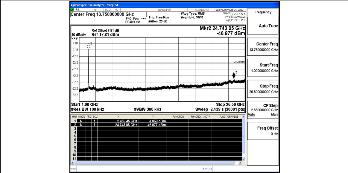
11G_Ant1_2462_1000~26500
