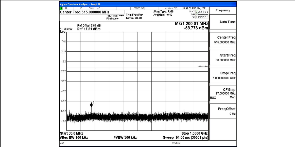
11B_Ant1_2462_30~1000
