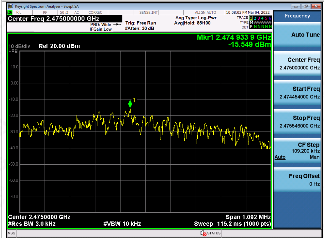
Test_Graph_GFSK_ANT1_2475_PSD
