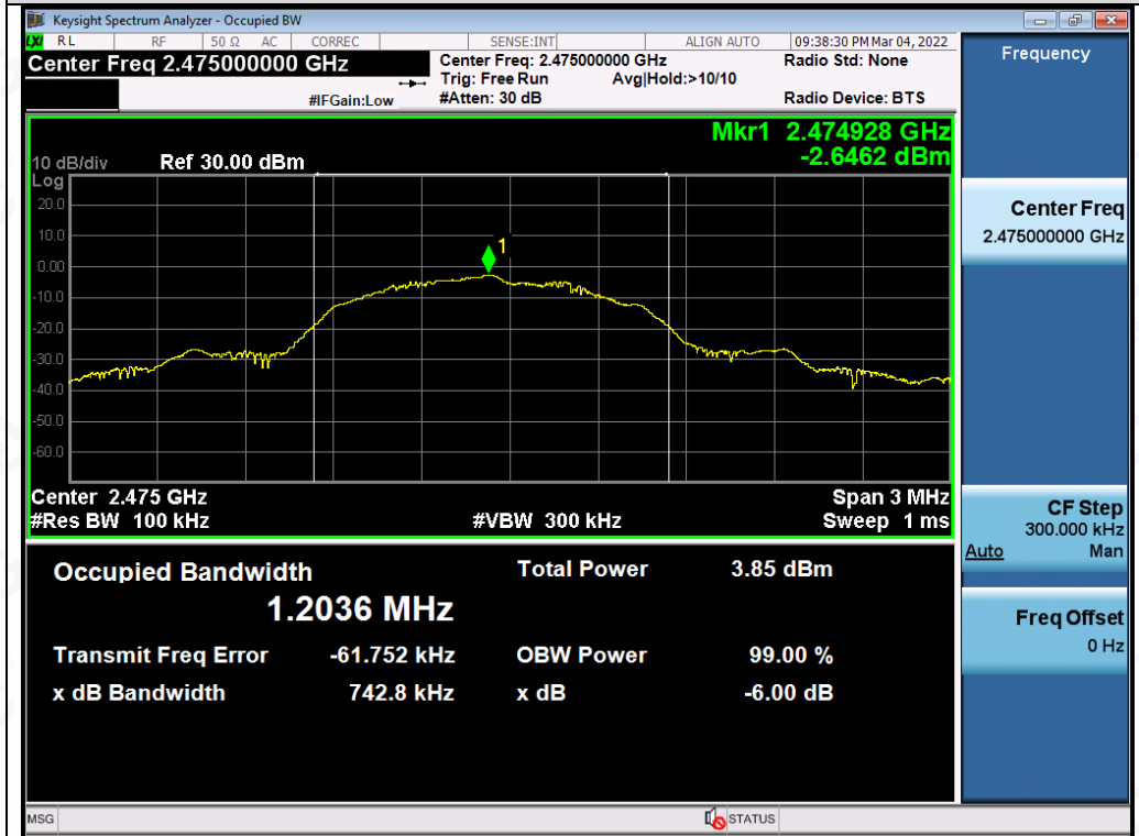
Test_Graph_GFSK_ANT1_2475_DTSBW
