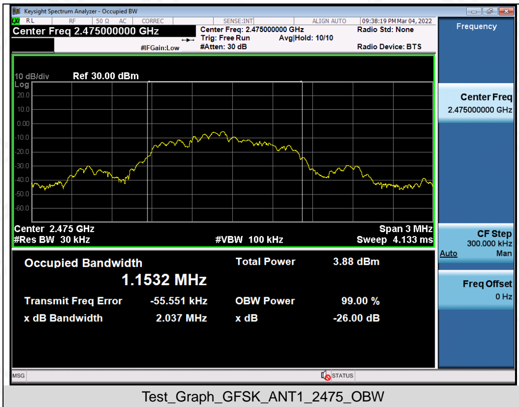
Test_Graph_GFSK_ANT1_2475_OBW
