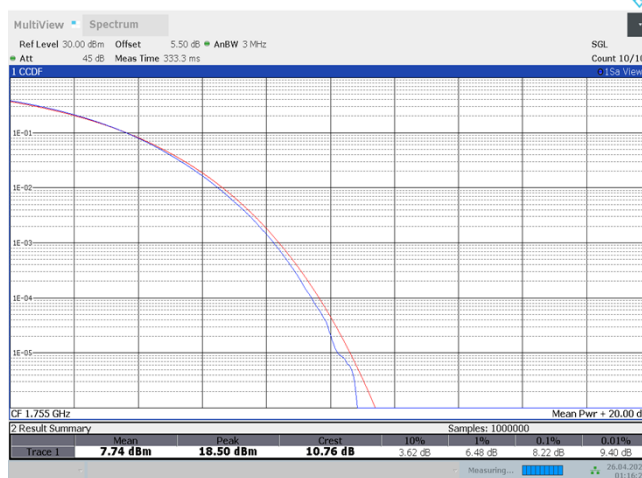
66-66-20MHz-20MHz-QPSK-QPSK-132323-132521-100RB#0-100RB#0
