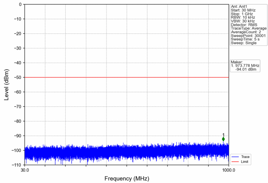
n48_30kHz_SISO_NTNV_40MHz_CP-OFDM_QPSK_3570MHz_Inner_1RB_Left
