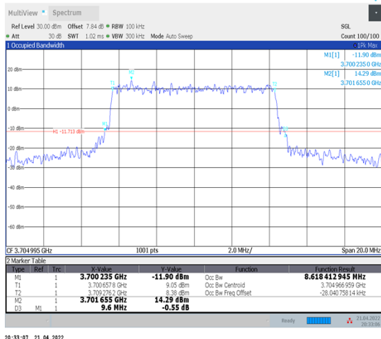
1-N78-3700-3800--30-10-L-1-DFT-QPSK-Outer_Full-24@0-Ant1-8.618-9.600-≤10-PASS
