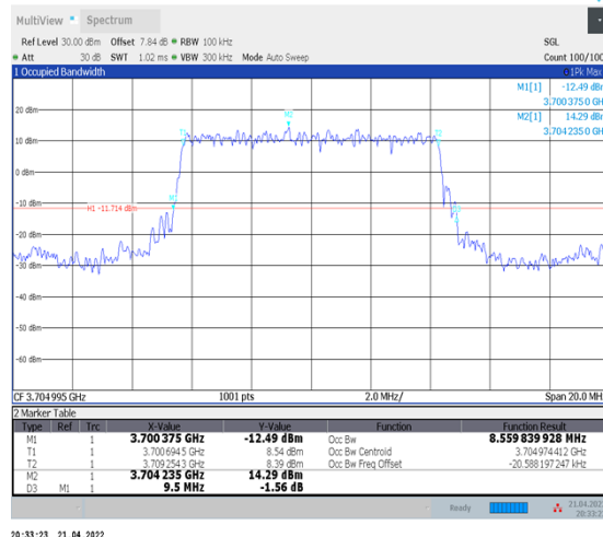
1-N78-3700-3800--30-10-L-2-DFT-PI2BPSK-Outer_Full-24@0-Ant1-8.56-9.500-≤10-PASS
