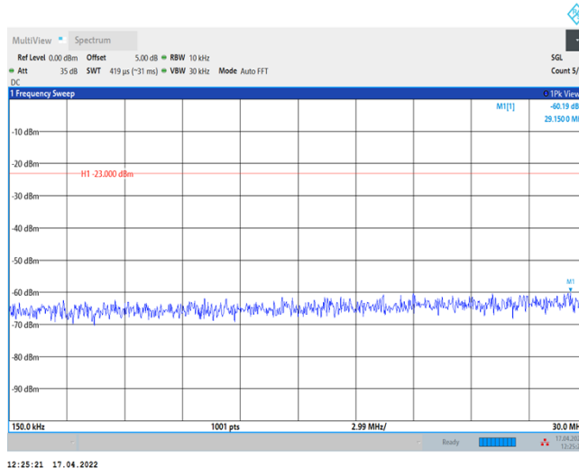
Band4-20MHz-QPSK-20050-1RB#0-Range2:0.15~30MHz
