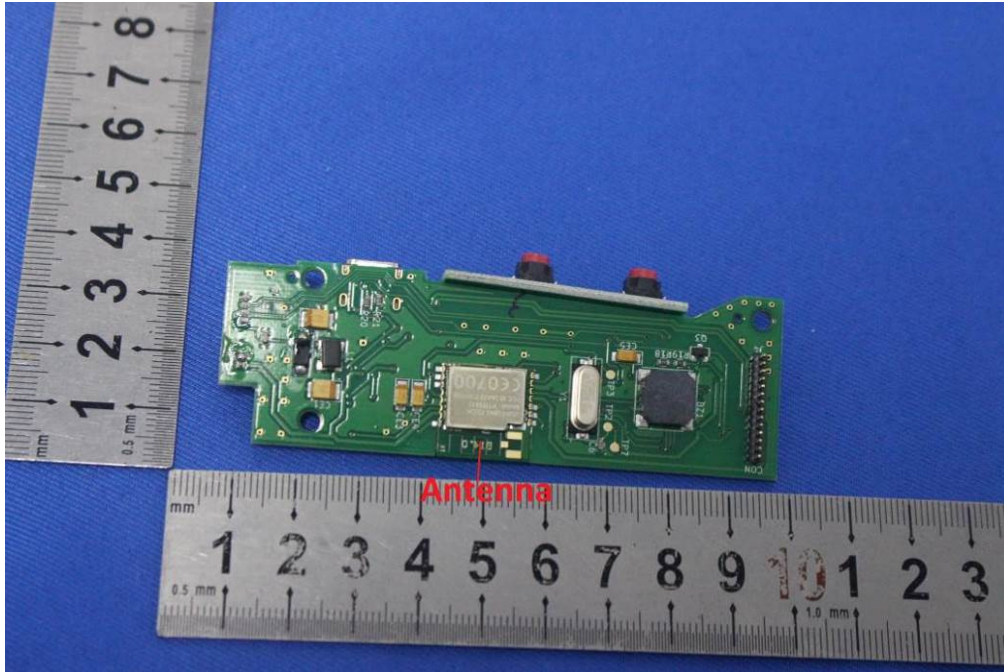
BLE Antenna
