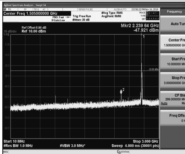
Band41_10MHz_QPSK_41190_1RB#0
