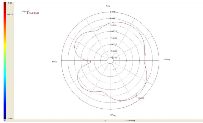
XY-Plane 2442MHz
