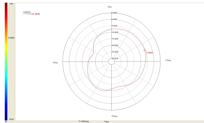
YZ-Plane 2442MHz
