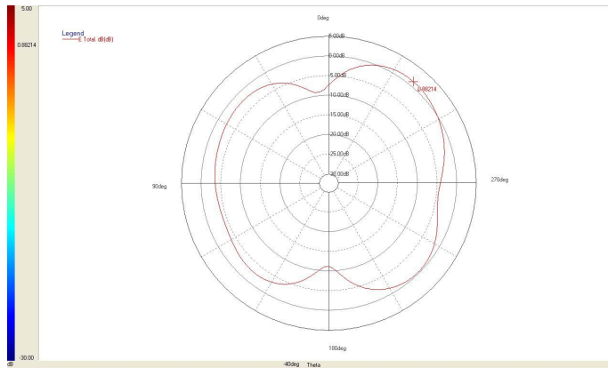
XZ-Plane 2442MHz
