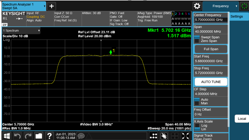
11AC20MIMO_Ant1_5700
