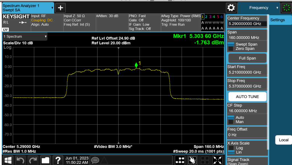
11AC80MIMO_Ant1_5290
