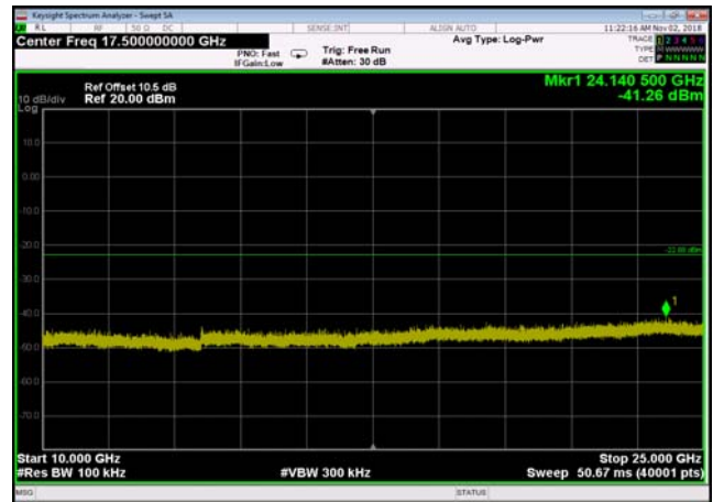
,Plot 5,10000MHz~25000MHz-802.11n(HT40),2452MHz
