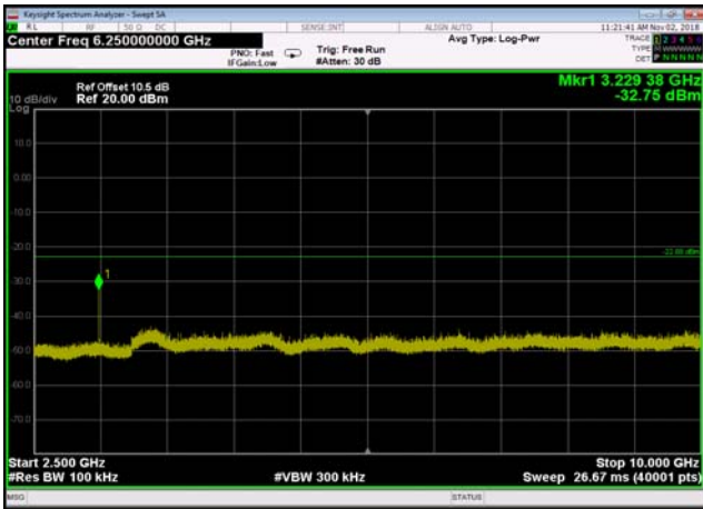
,Plot 4,2500MHz~10000MHz-802.11n(HT40),2452MHz
