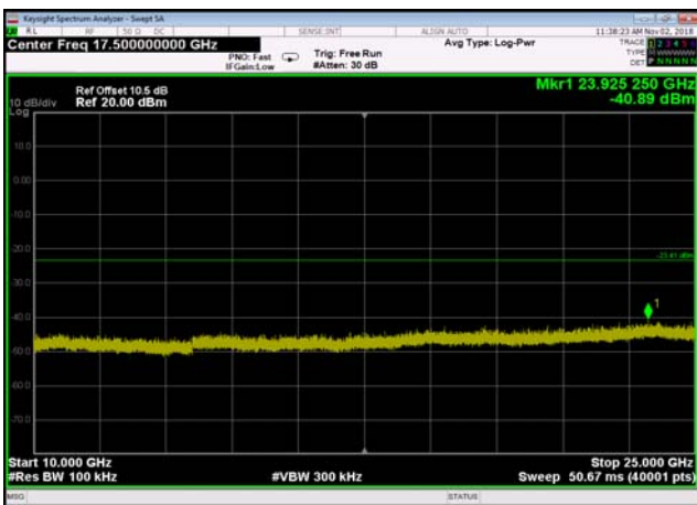
,Plot 5,10000MHz~25000MHz-802.11n(HT40),2437MHz
