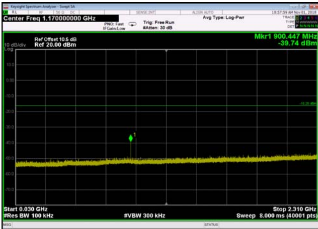
,Plot 3,30MHz~2310MHz-802.11b,2462MHz
