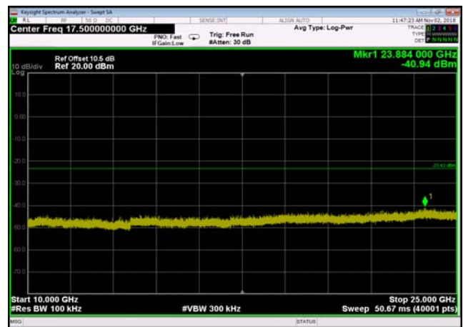
,Plot 5,10000MHz~25000MHz-802.11n(HT40),2452MHz
