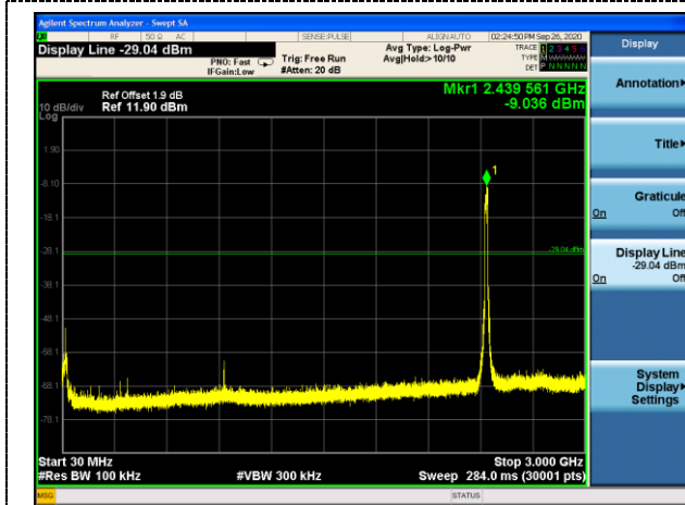
30MHz-3GHz
