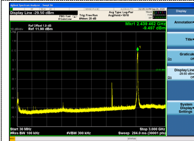
30MHz-3GHz
