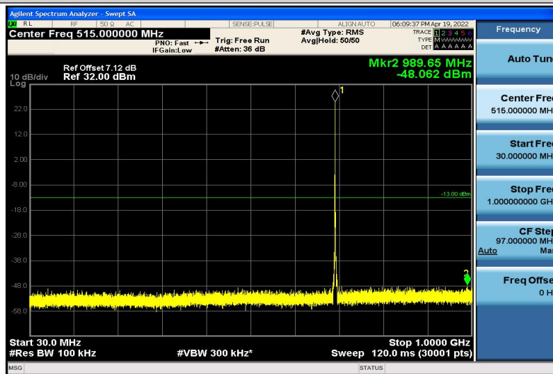
Band12-1.4MHz-QPSK-23017-1RB#0-30~1000MHz
