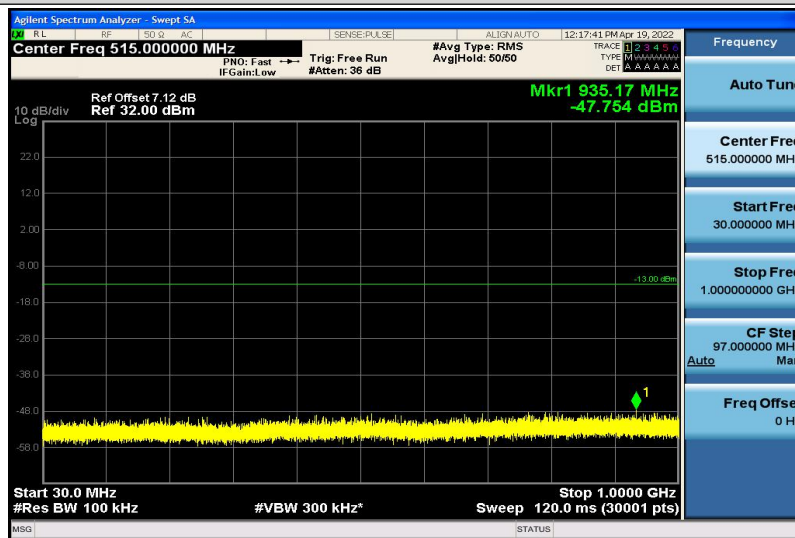
Band2-20MHz-QPSK-18700-1RB#0-30~1000MHz
