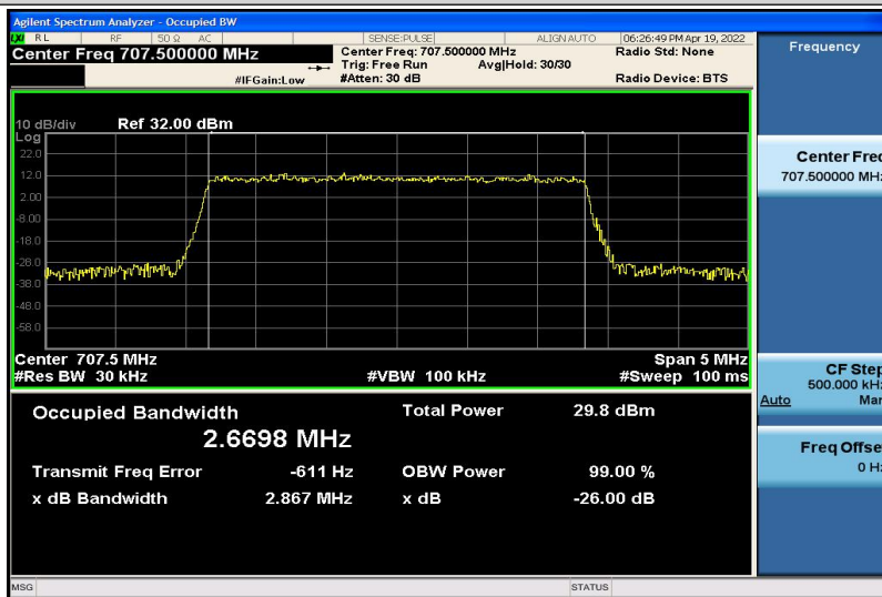
Band12-3MHz-16QAM-23095-15RB#0-2.6698
