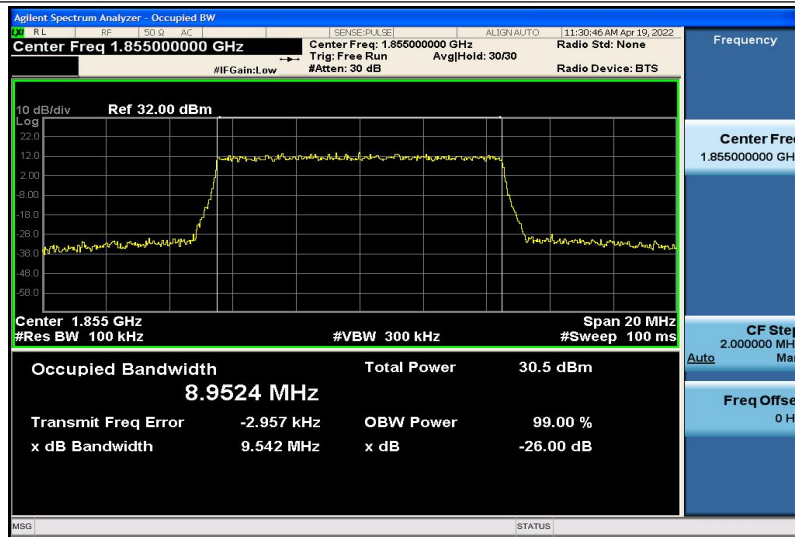
Band2-10MHz-QPSK-18650-50RB#0-8.9524
