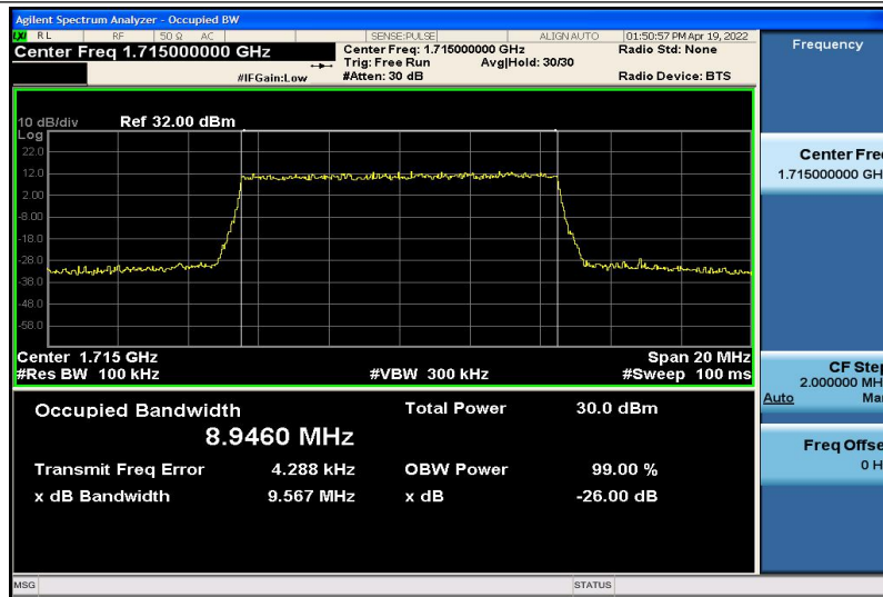
Band4-10MHz-QPSK-20000-50RB#0-8.9460
