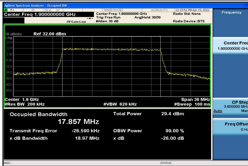
Band2-20MHz-16QAM-19100-100RB#0-17.857
