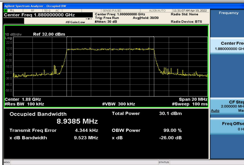
Band2-10MHz-QPSK-18900-50RB#0-8.9385
