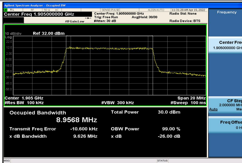
Band2-10MHz-QPSK-19150-50RB#0-8.9568
