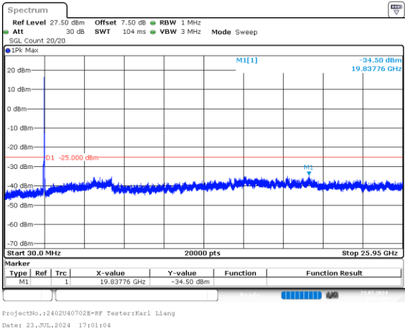
20MHz_Middle_QPSK_100@0 -34.50dBm
