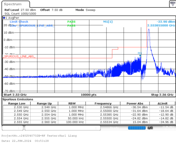
3_5MHz_Low_QPSK_1@0
