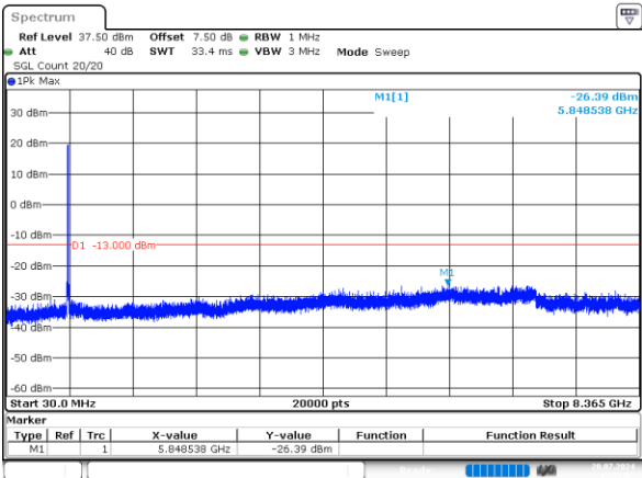
10MHz_Middle_QPSK_50@0 -26.39dBm
