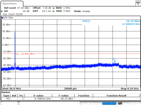
10MHz_Low_QPSK_50@0 -26.10dBm
