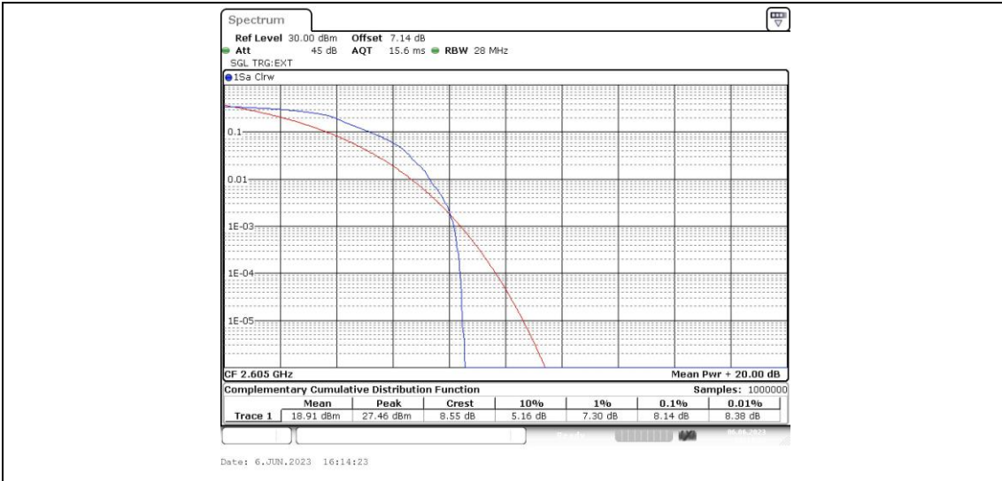
Band41-10MHz-QPSK-40740-50RB#0
