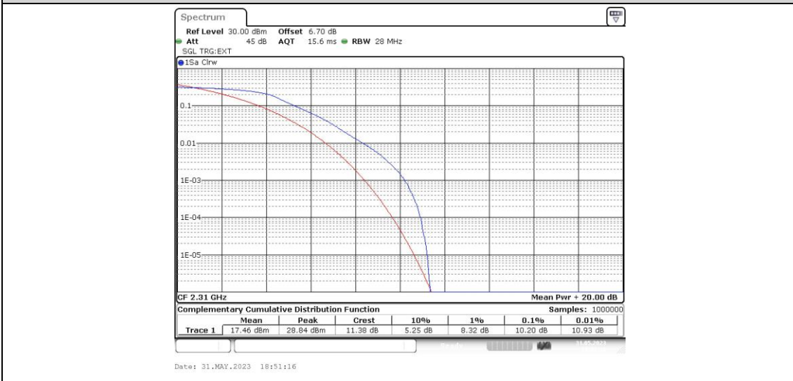
Band40-5MHz-QPSK-38775-1RB#0
