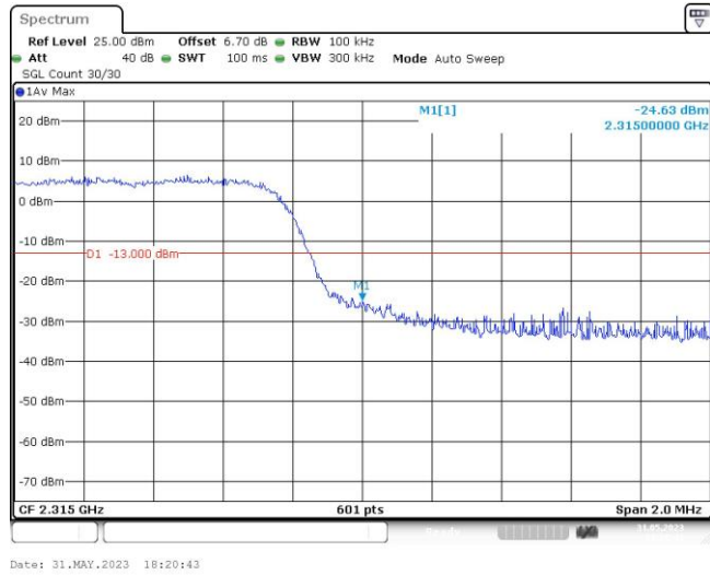
Band40-10MHz-QPSK-38750-1RB#0
