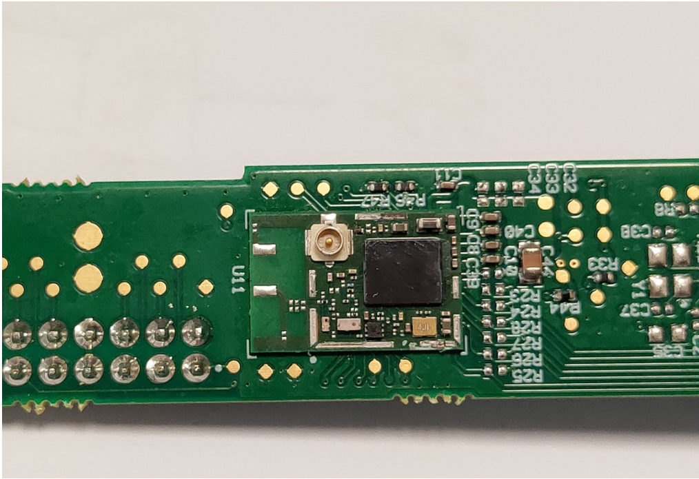
Pic 11. RF module
