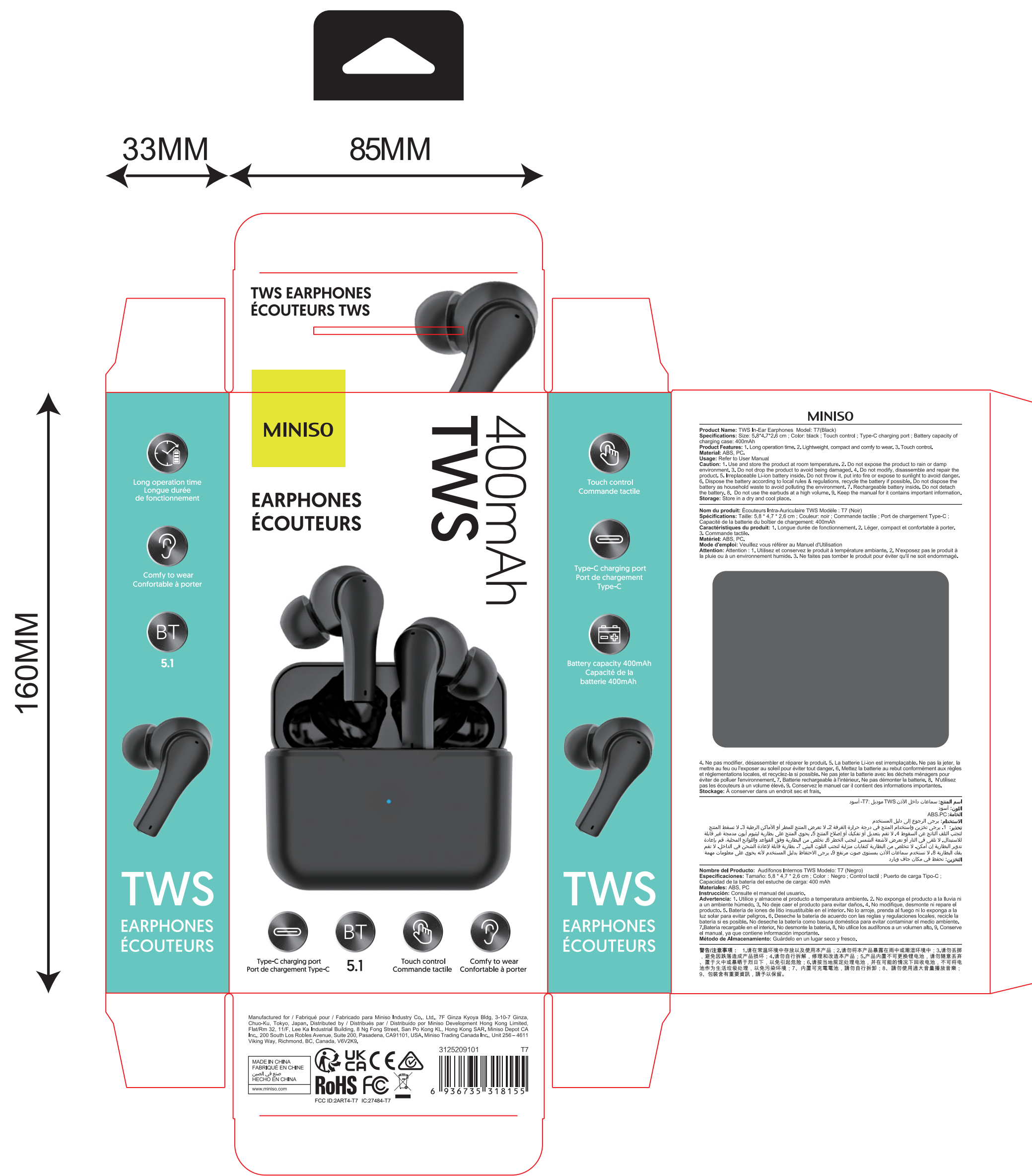
TWS入耳式耳机 型号:T7(黑色)
