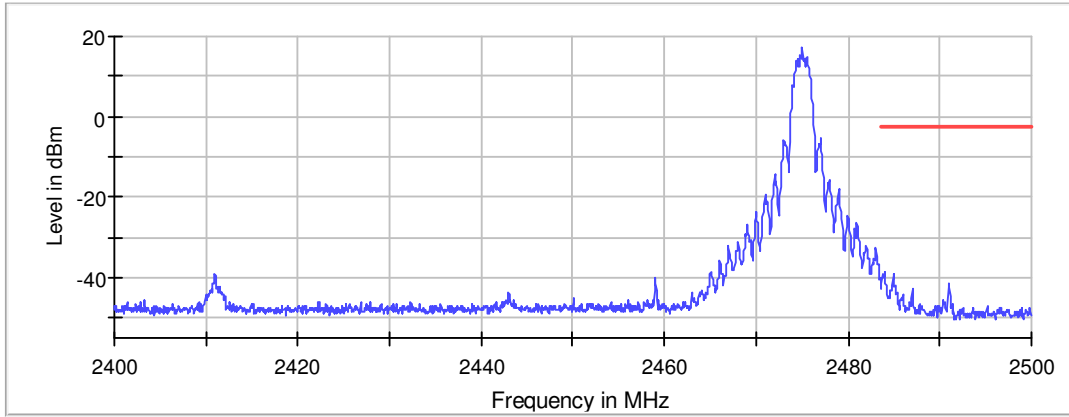
Band Edge
