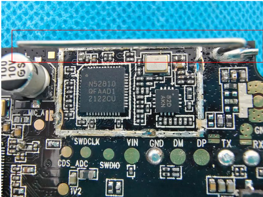
FHSS Antenna
