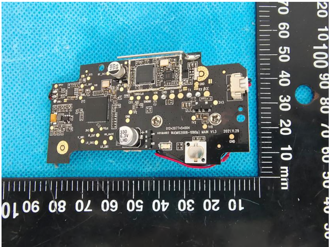
FHSS Antenna
