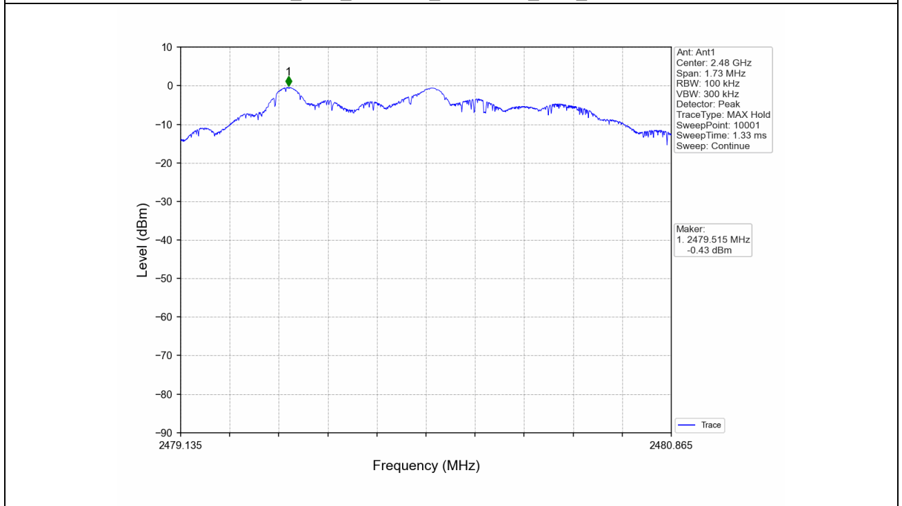
2M_HCH_2480MHz_DataRate=_Ant1_NTNV
