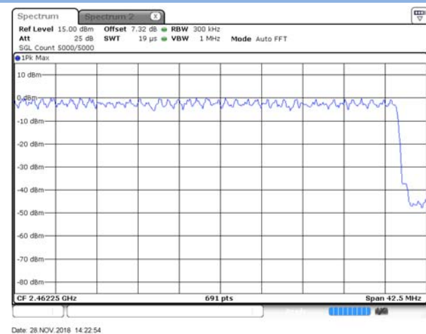
\Pi/4 -DQPSK 2.4415 GHz ~ 2.4835 GHz
