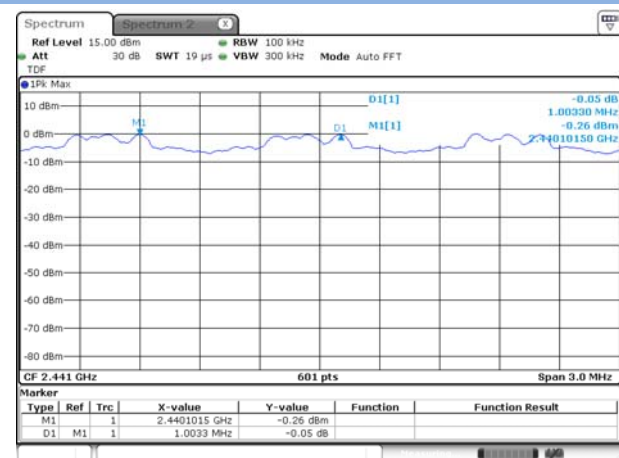
\Pi/4 -DQPSK
