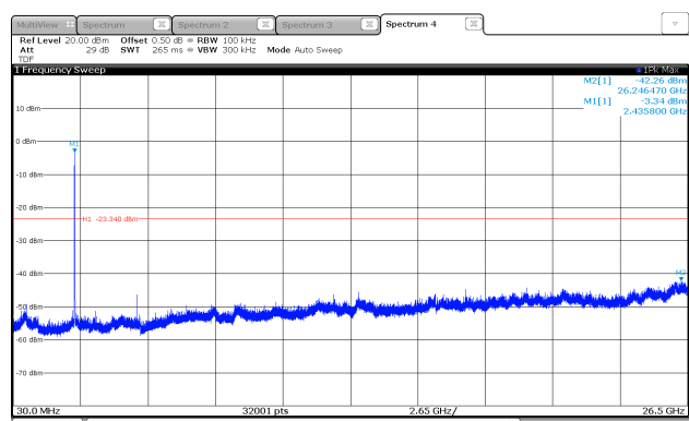
802.11b / 6 ch
