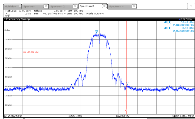
802.11b / 11 ch
