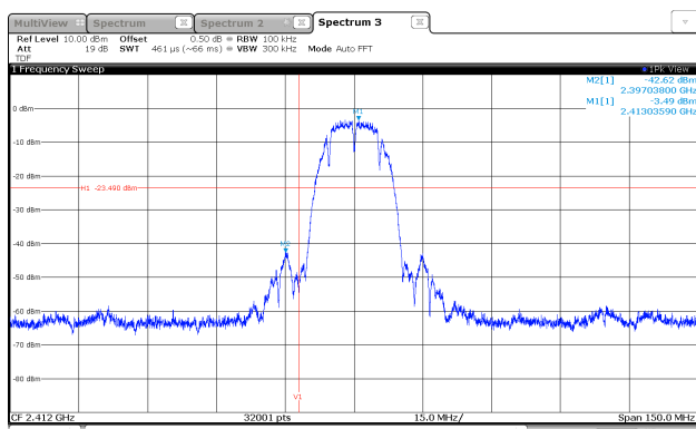
802.11b / 1 ch
