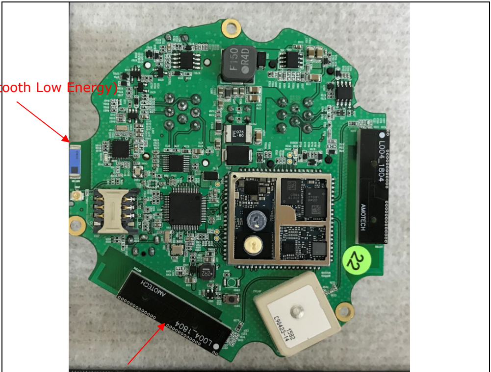
Chip Antenna (LTE, WCDMA)
