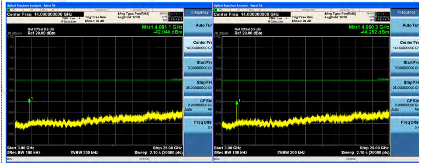
3GHz-25GHz
