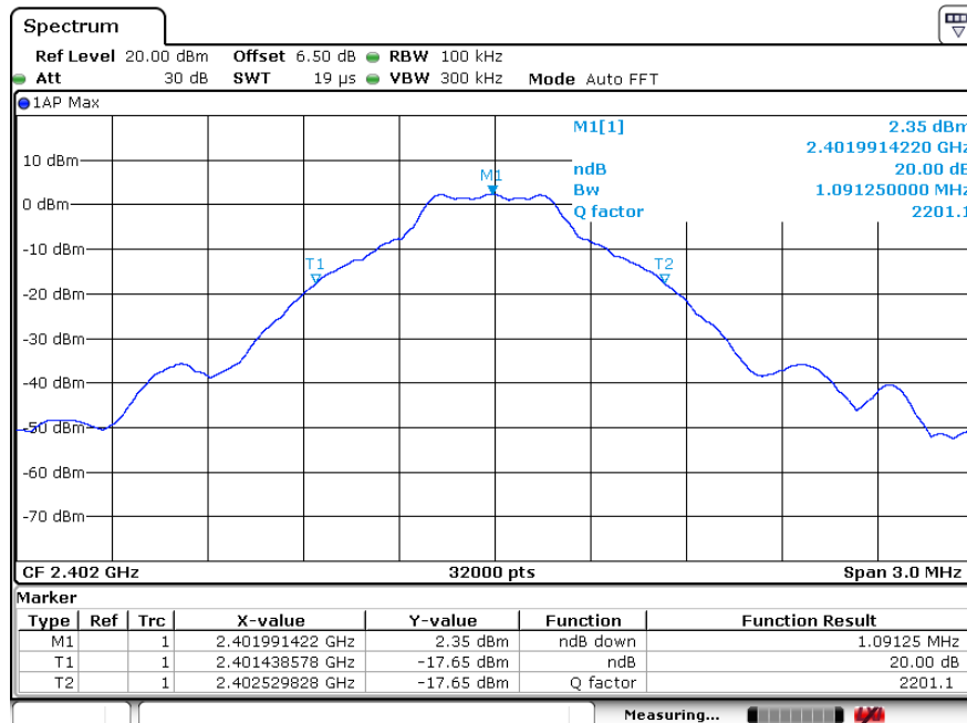
GFSK 2402MHZ
