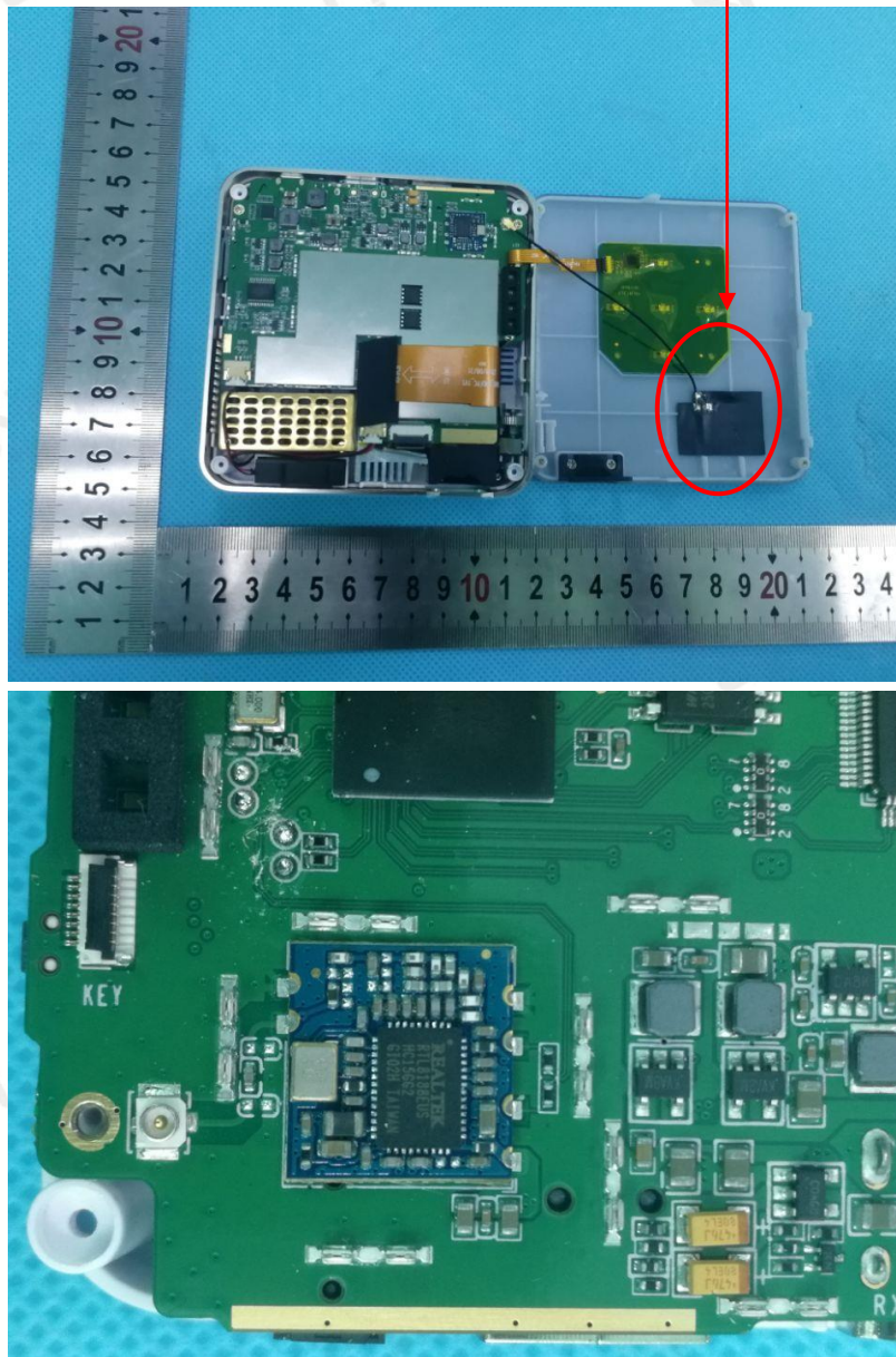
ANTENNA
