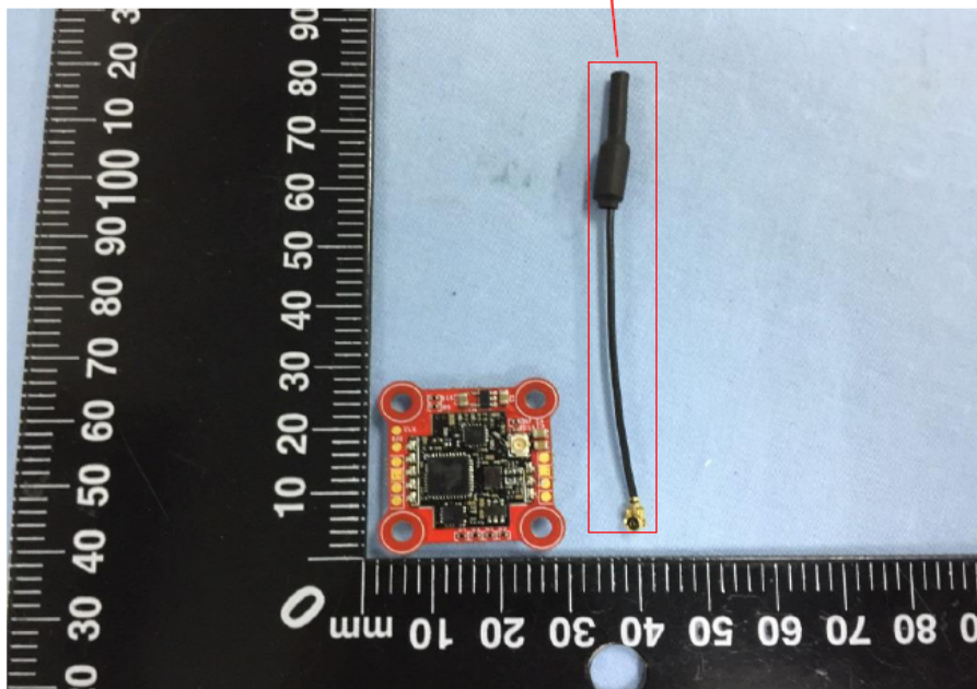
5.8G Antenna
