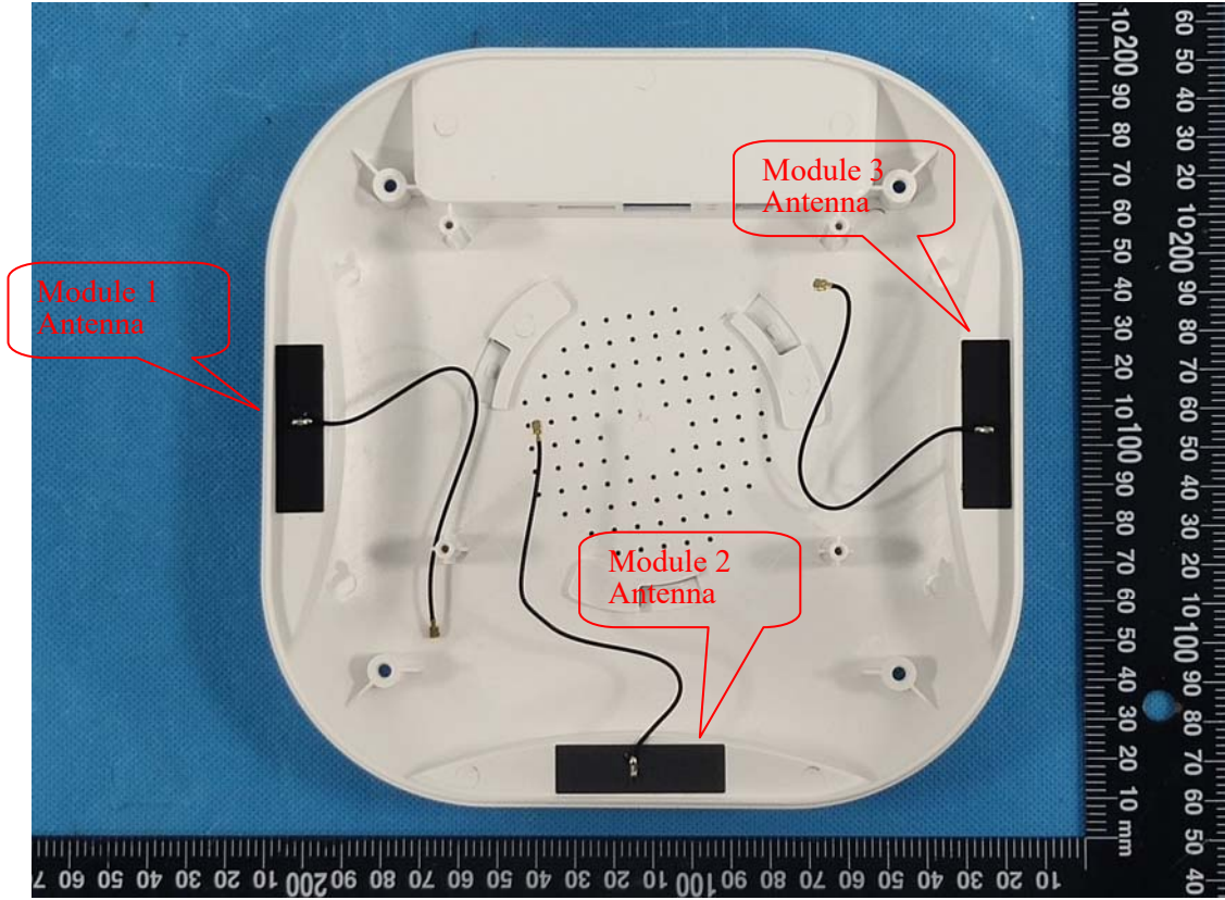
Module 3 Antenna
