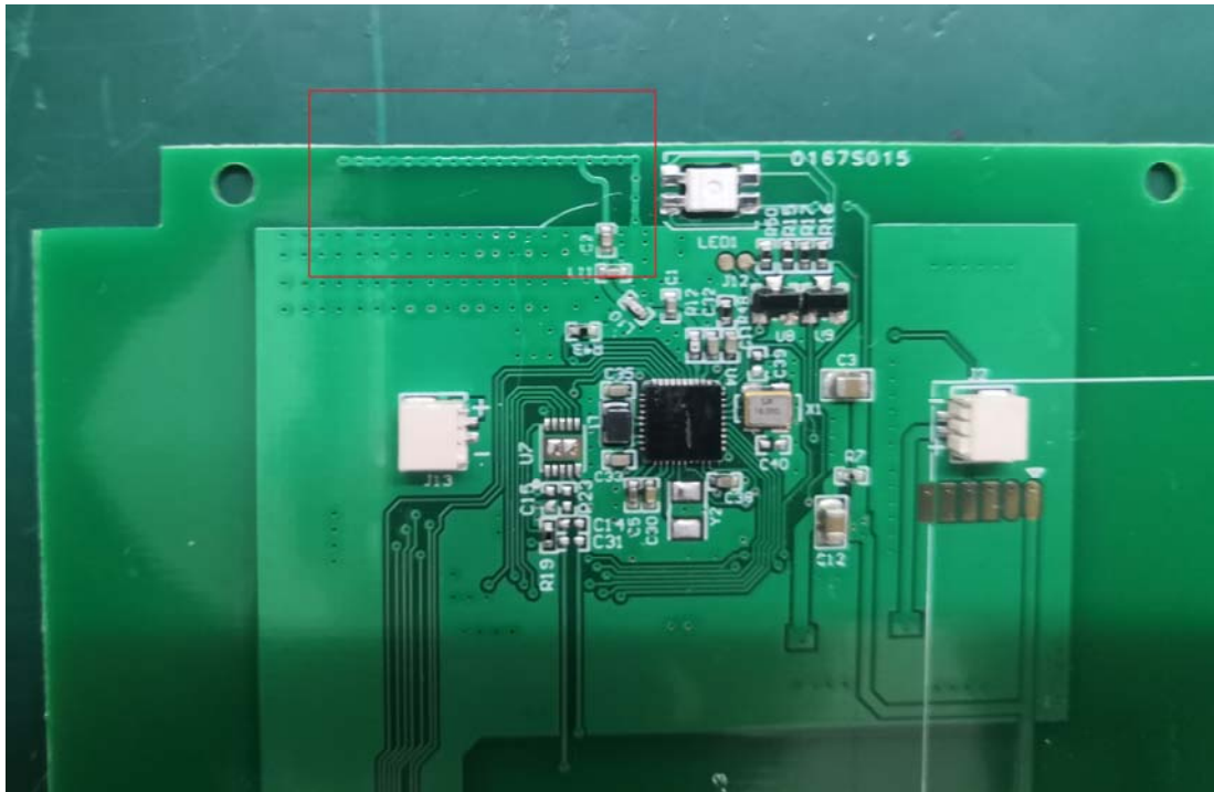
Antenna
