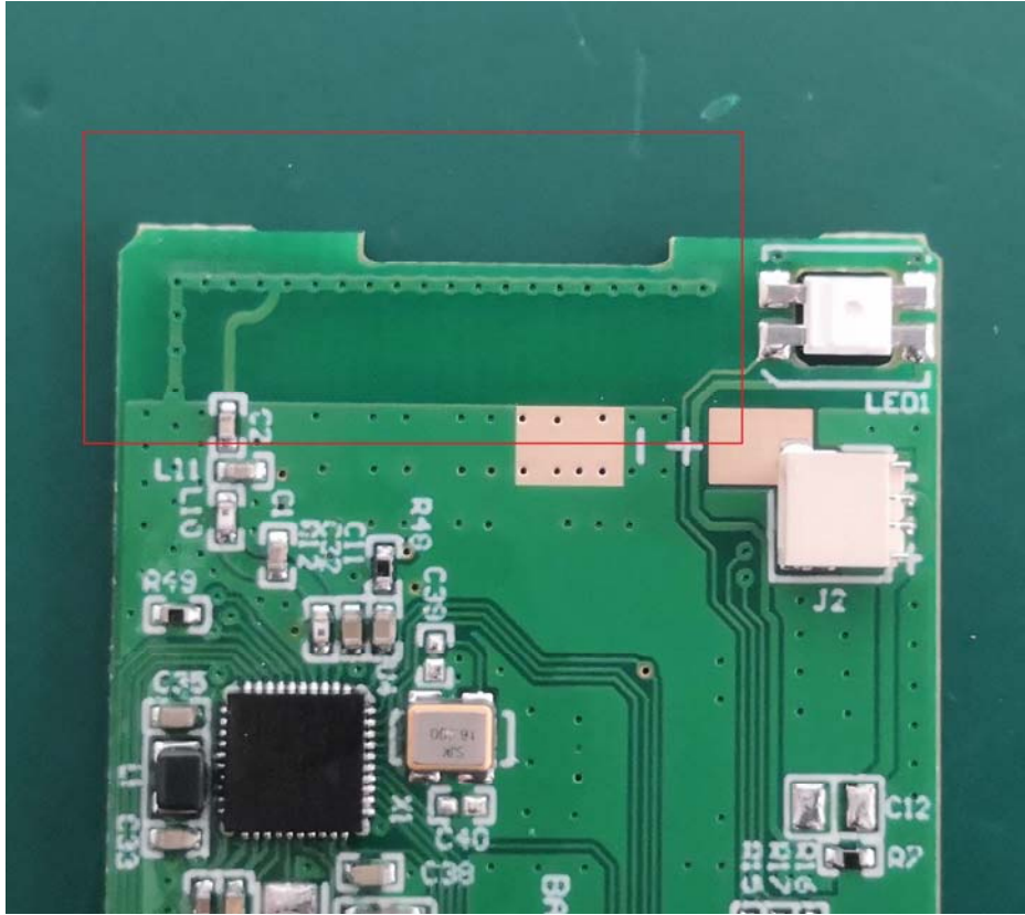
Antenna
