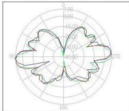
E-Plane
