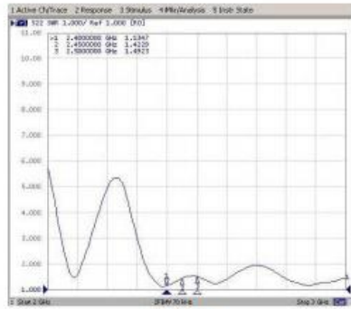
V.S.W.R
