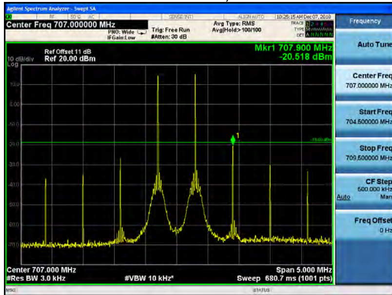
AGC+10dB, UL
