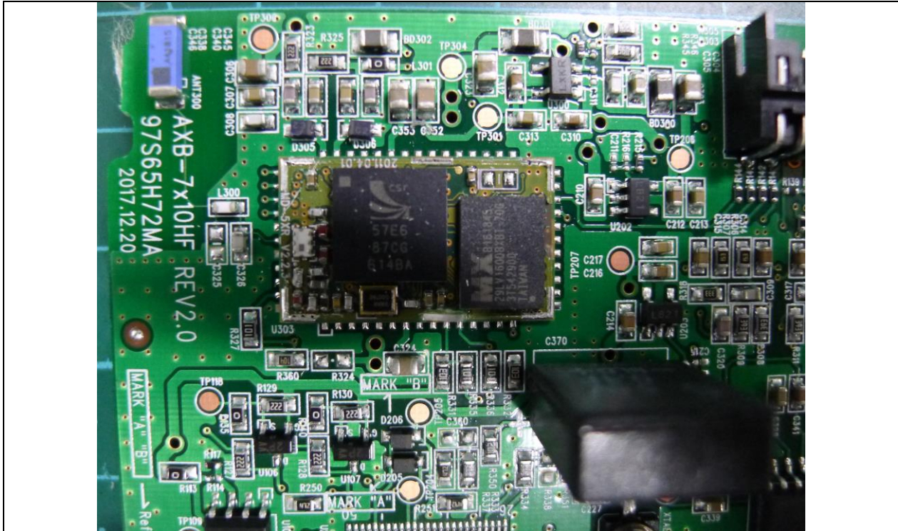
Bluetooth Module
