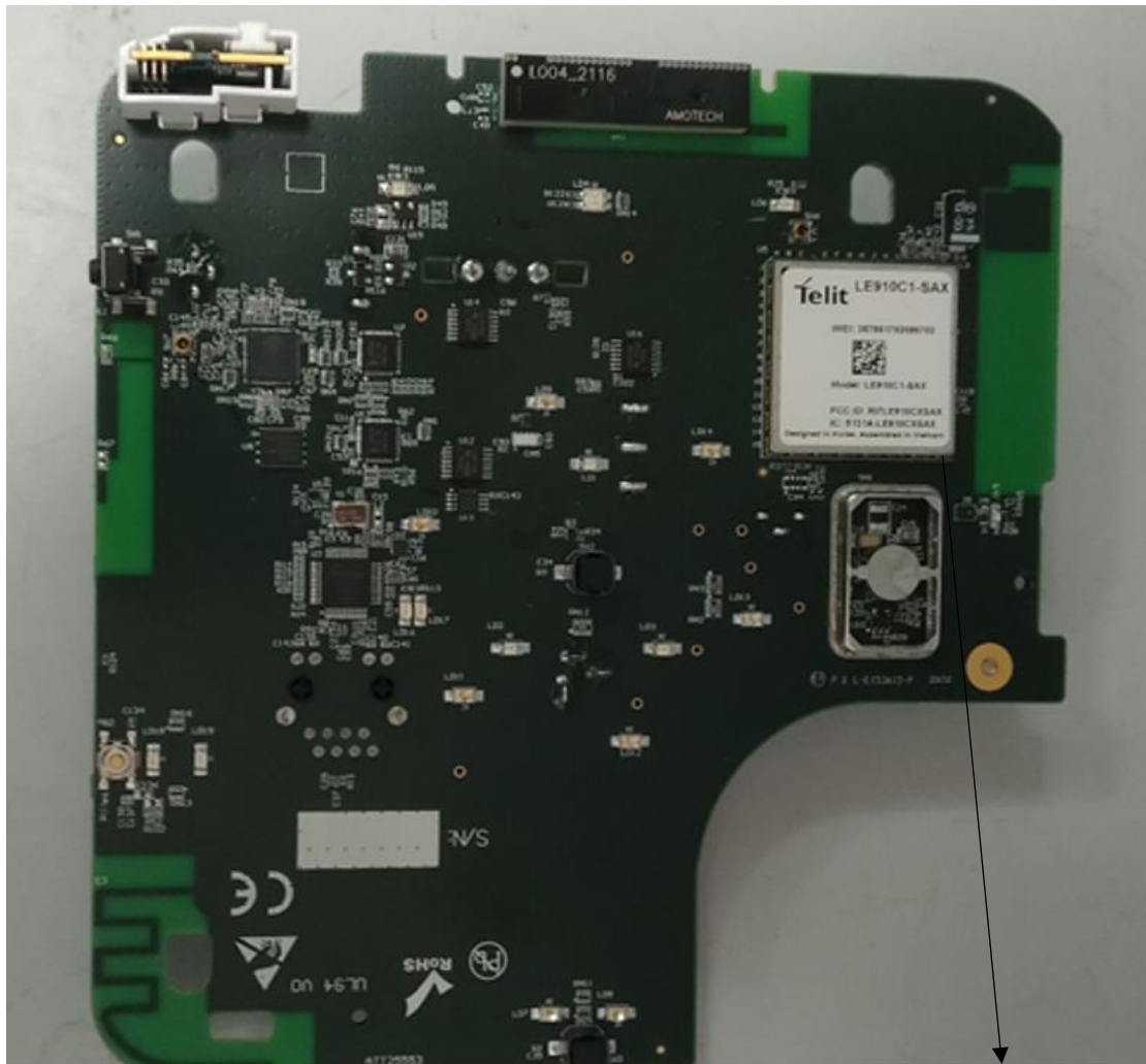
RI7LE910CXSA module
