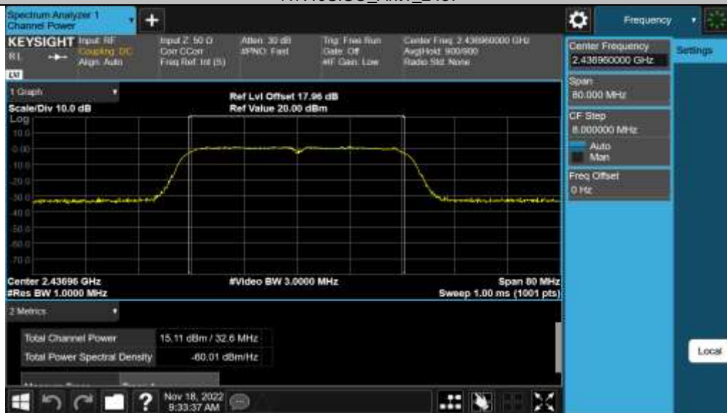
11N40SISO_Ant1_2437
