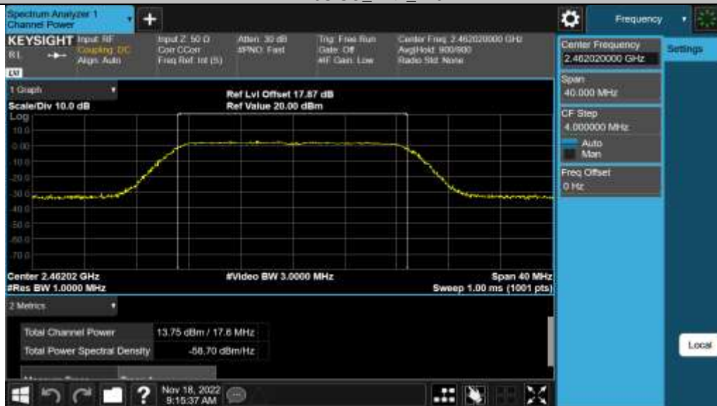
11N20SISO_Ant1_2462
