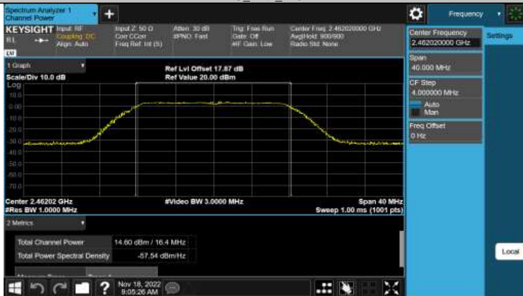
11G_Ant1_2462
