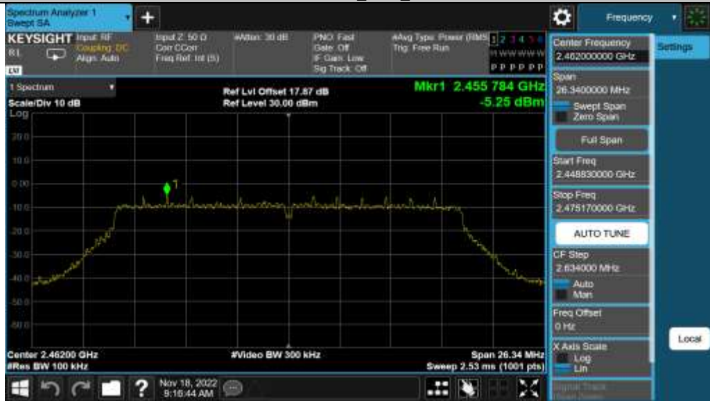
11N20SISO_Ant1_2462
