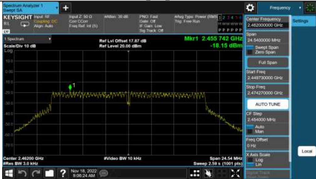
11G_Ant1_2462
