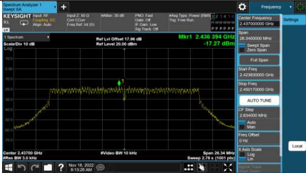
11N20SISO_Ant1_2437
