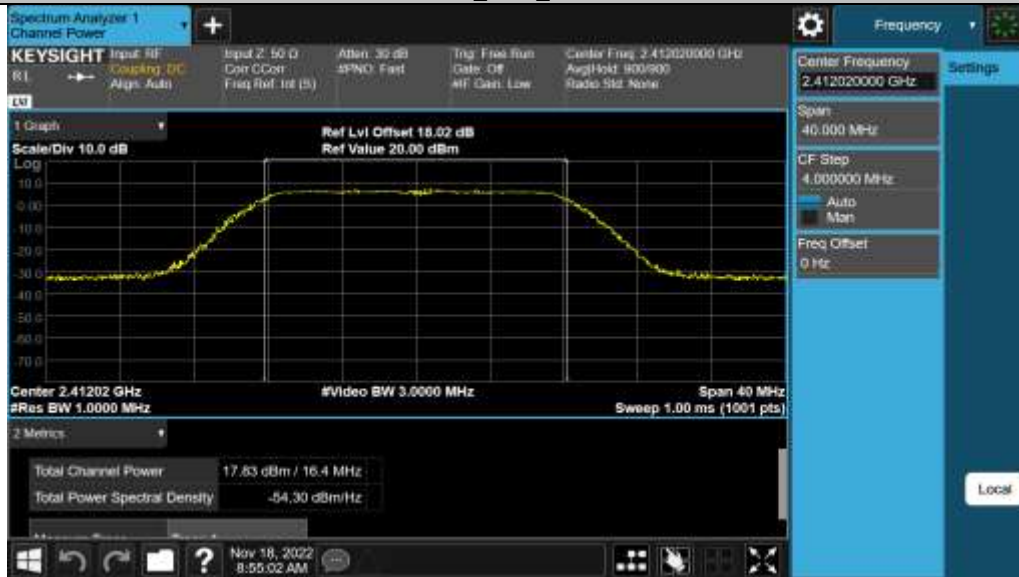
11G_Ant1_2412
