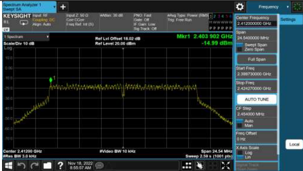
11G_Ant1_2412
