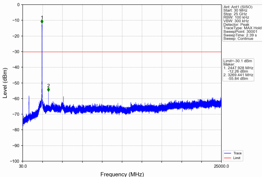
802.11n(HT40)_HCH_2452MHz_Ant1 (SISO)_NTNV
