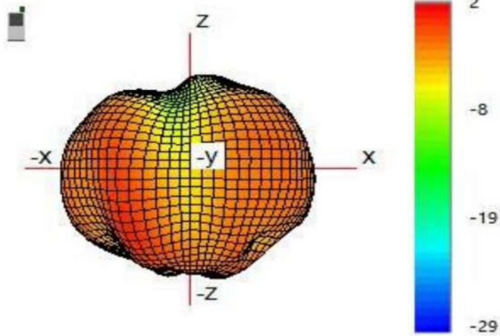
(4) 2.4GHz 的 3D 方向图(单位: dBi):
