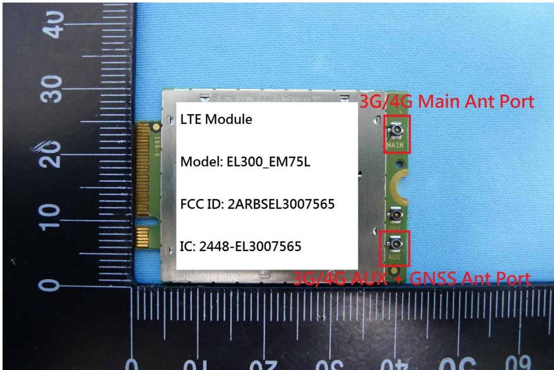
(64) RF Module (SIERRA EM7565)
