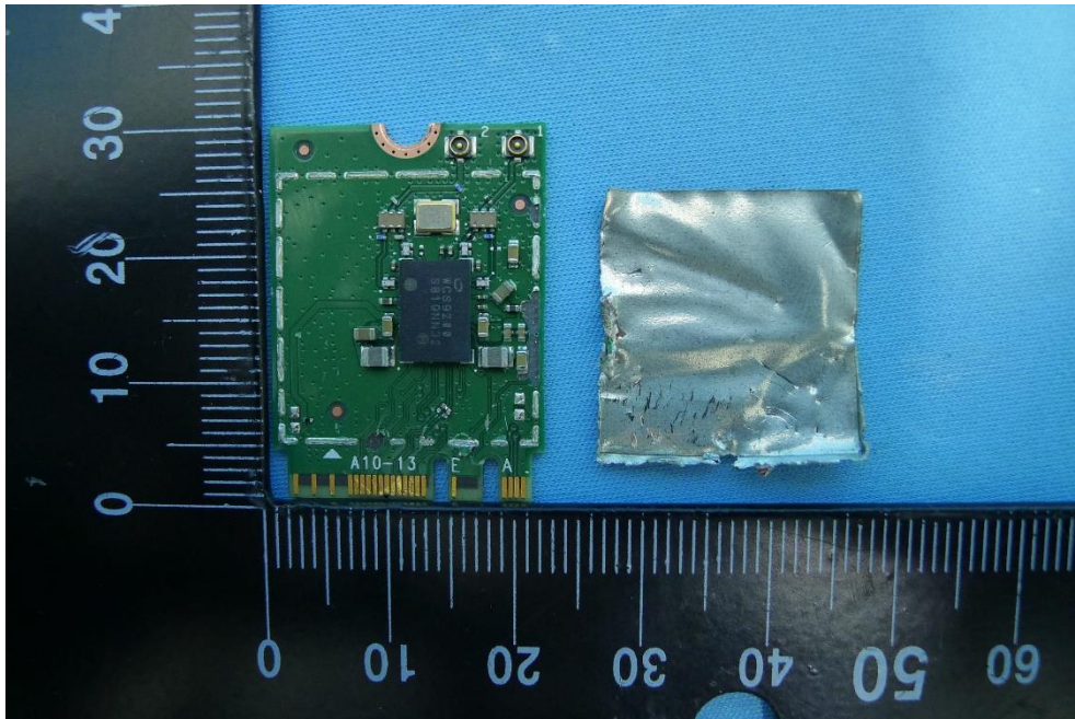
(60) RF Module (INTEL 9260NGW)
