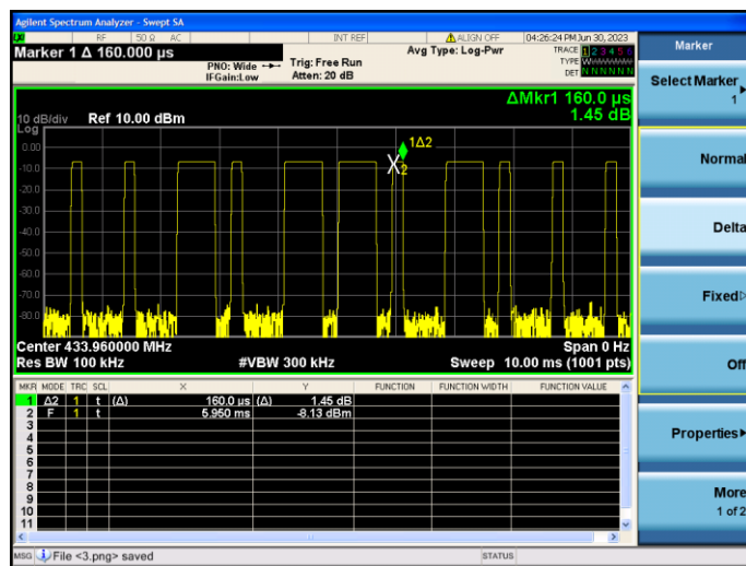
(Time per burst: 0.160 \text{ ms} * 13 \text{ pcs} )
