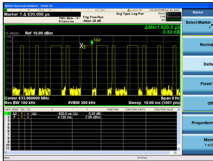
(Time per burst: 0.620 \text{ ms} * 12 \text{ pcs} )
