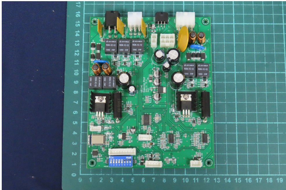
(31) EUT Photo
