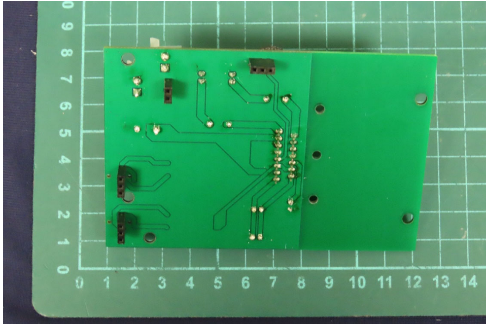
(41) EUT Photo
