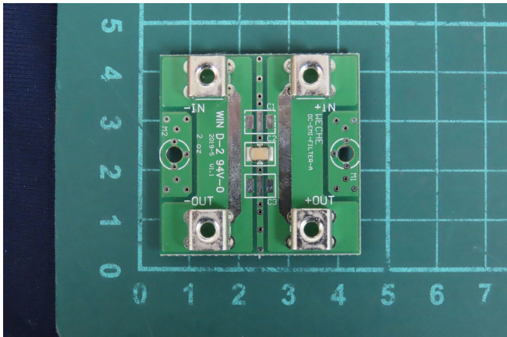
(12) EUT Photo
