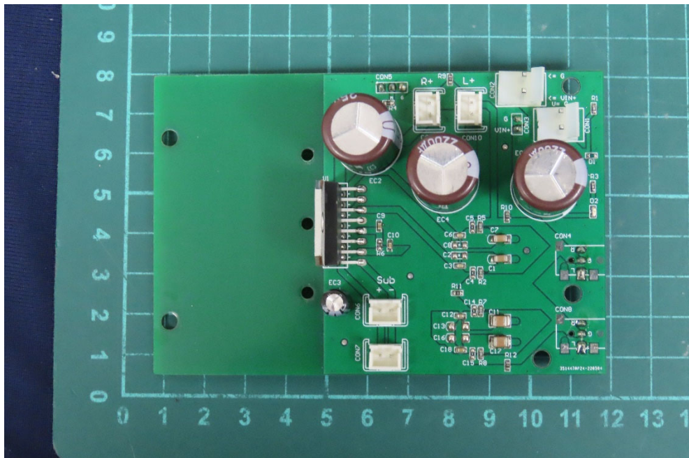
(40) EUT Photo
