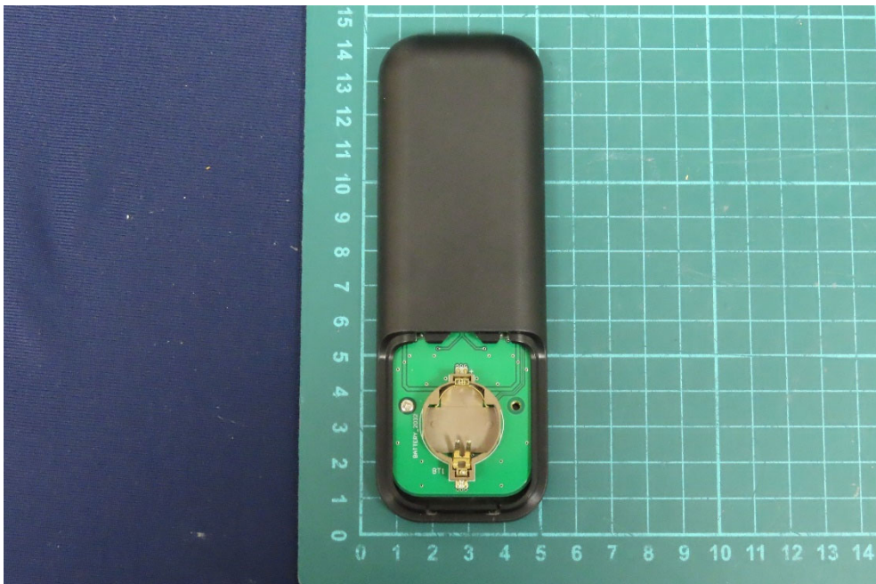
(56) EUT Photo
