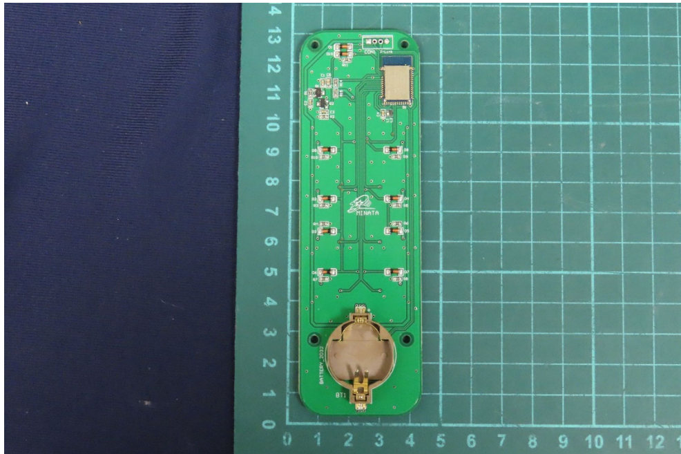
(61) EUT Photo
