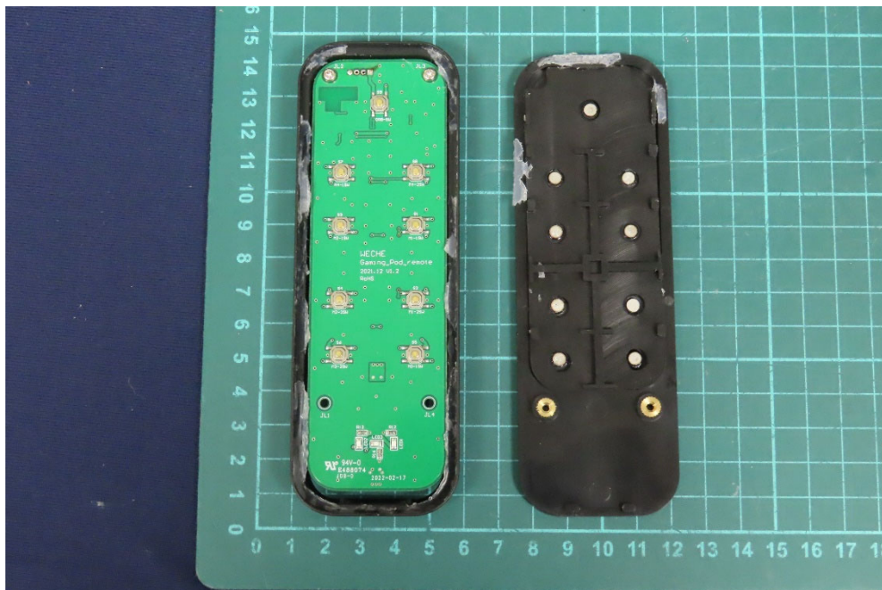
(57) EUT Photo
