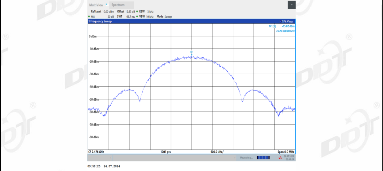
2.4G SRD_Ant2_2476
