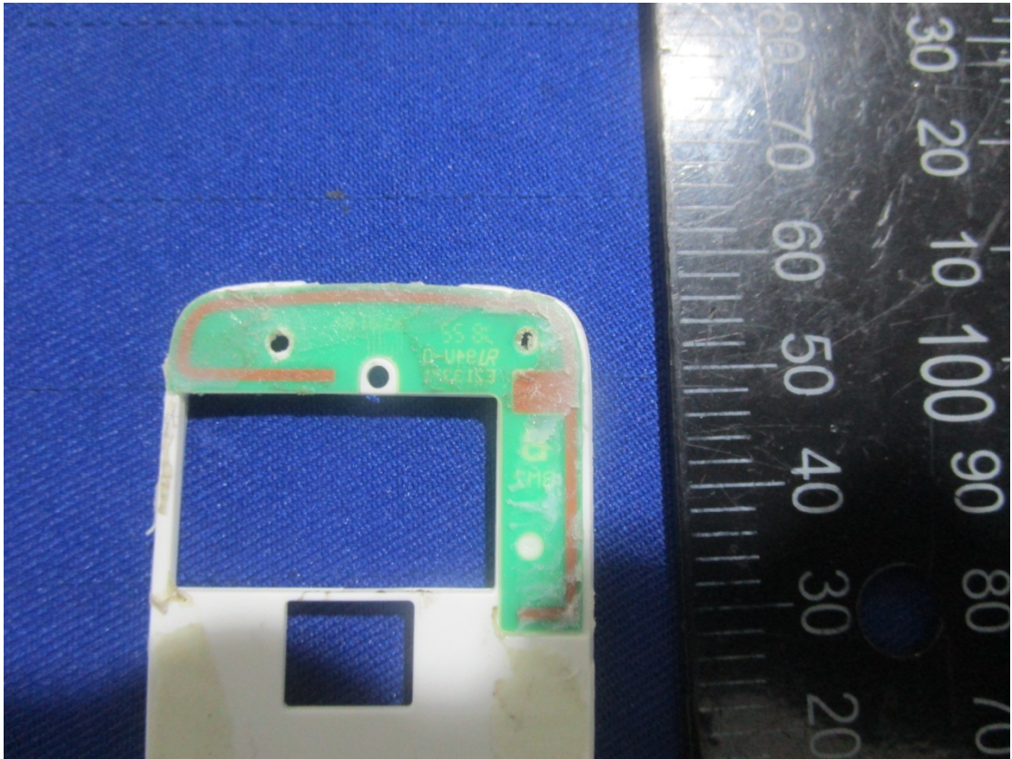
GSM Antenna
