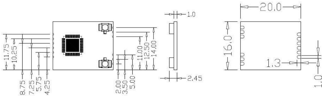
模组主视图
